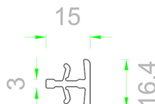
563/11 Mini Coupling
