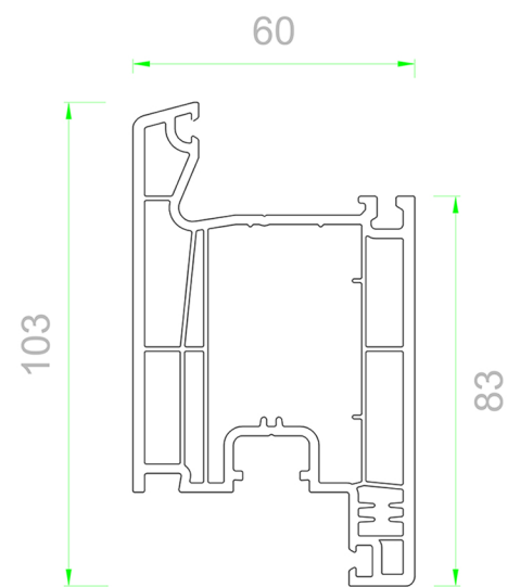
407/21 Door Sash
