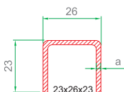
S-563TRE05 = S-507TRE05
